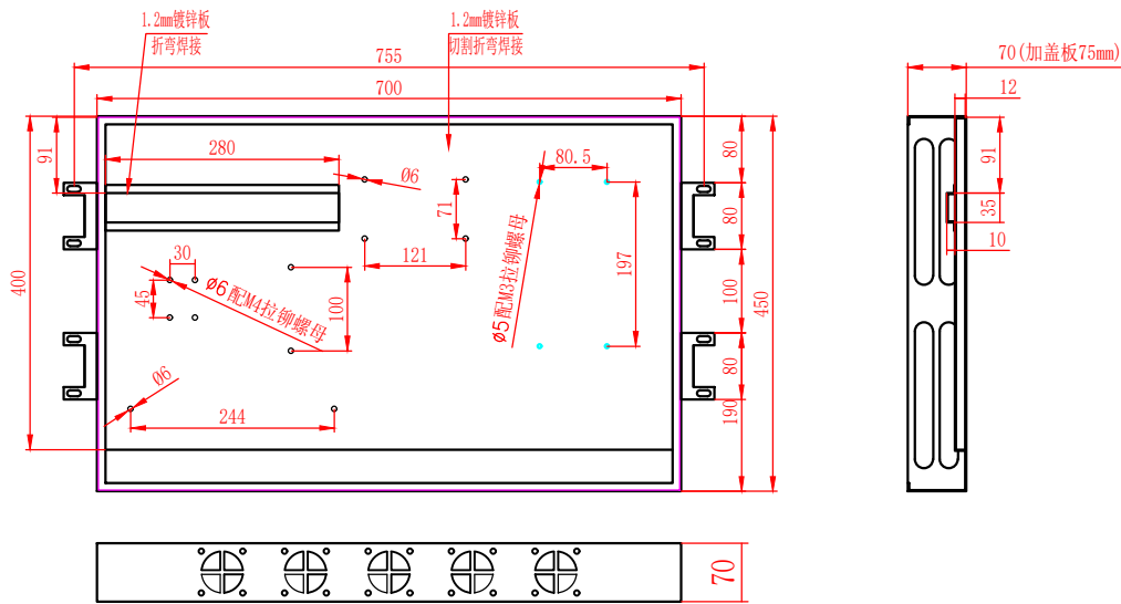
电气柜固定脚位置图
